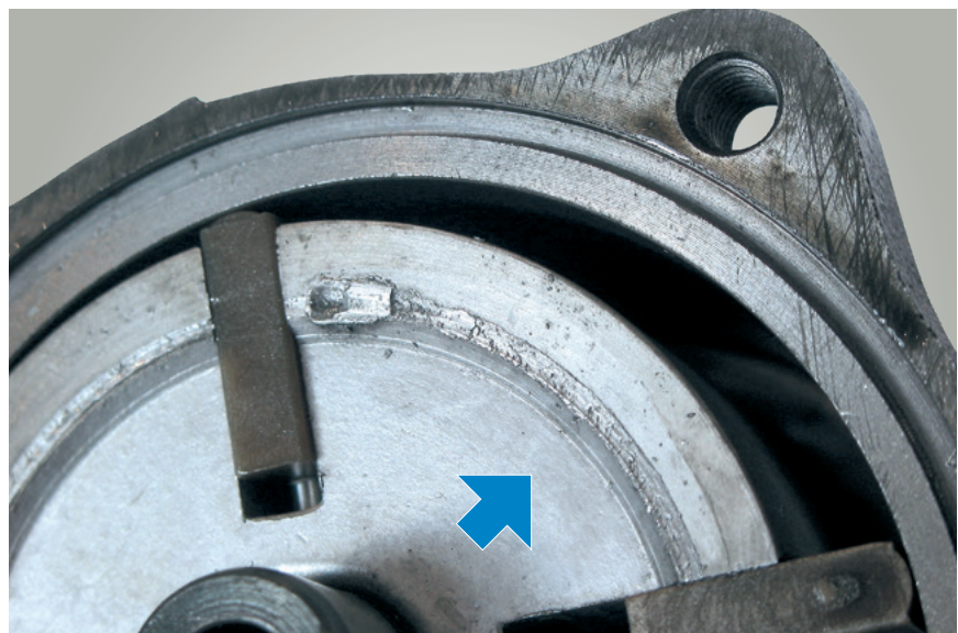
Esta bomba celular de paletas se ha „agarrotado“ por falta de aceite.
